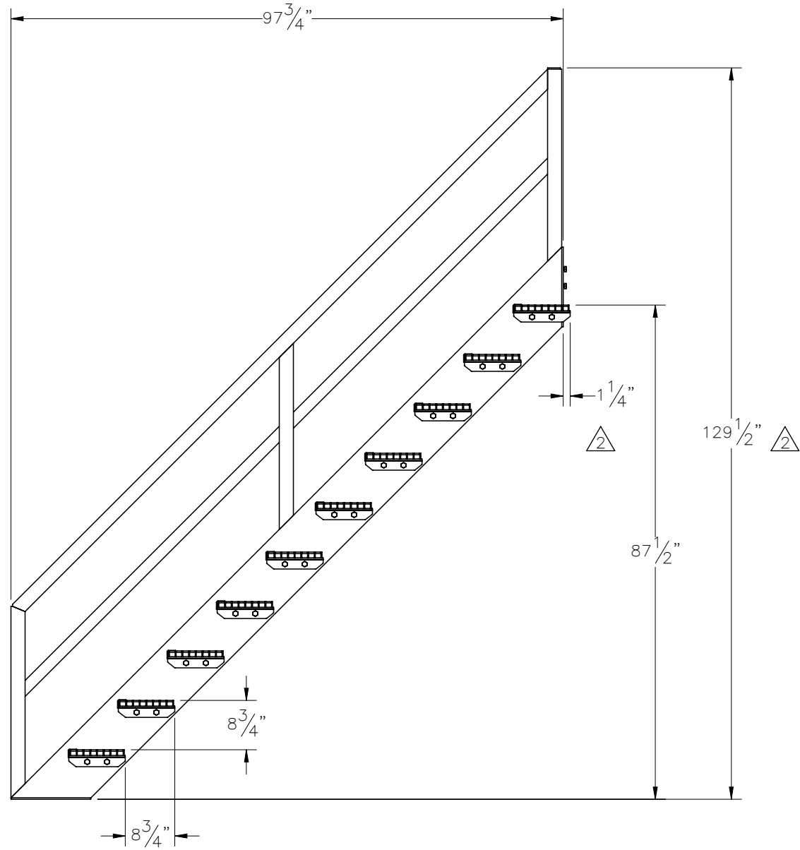
SECTION A-A
