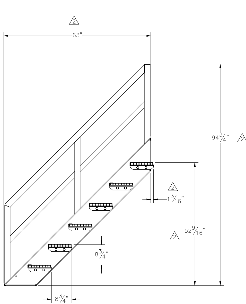
SECTION A-A
